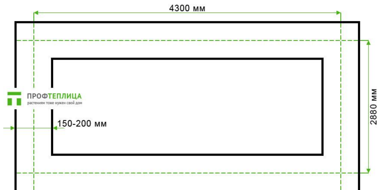
Размеры фундамента по осям и толщина стенок (вид сверху)
