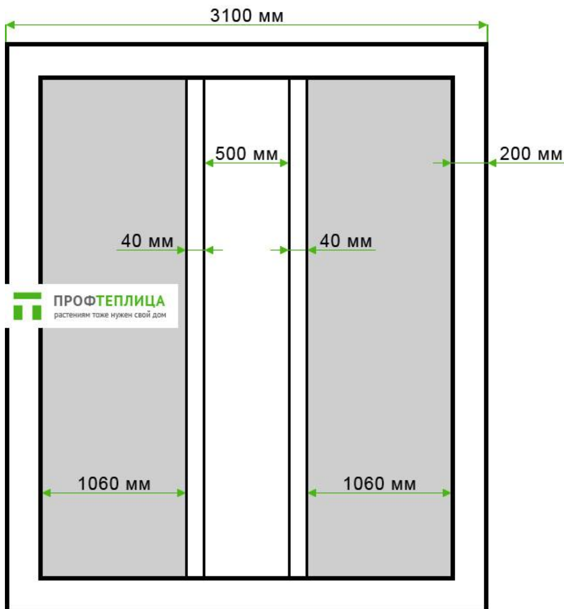
Вариант внутренней планировки теплицы «АСГ-12» (вид сверху)
