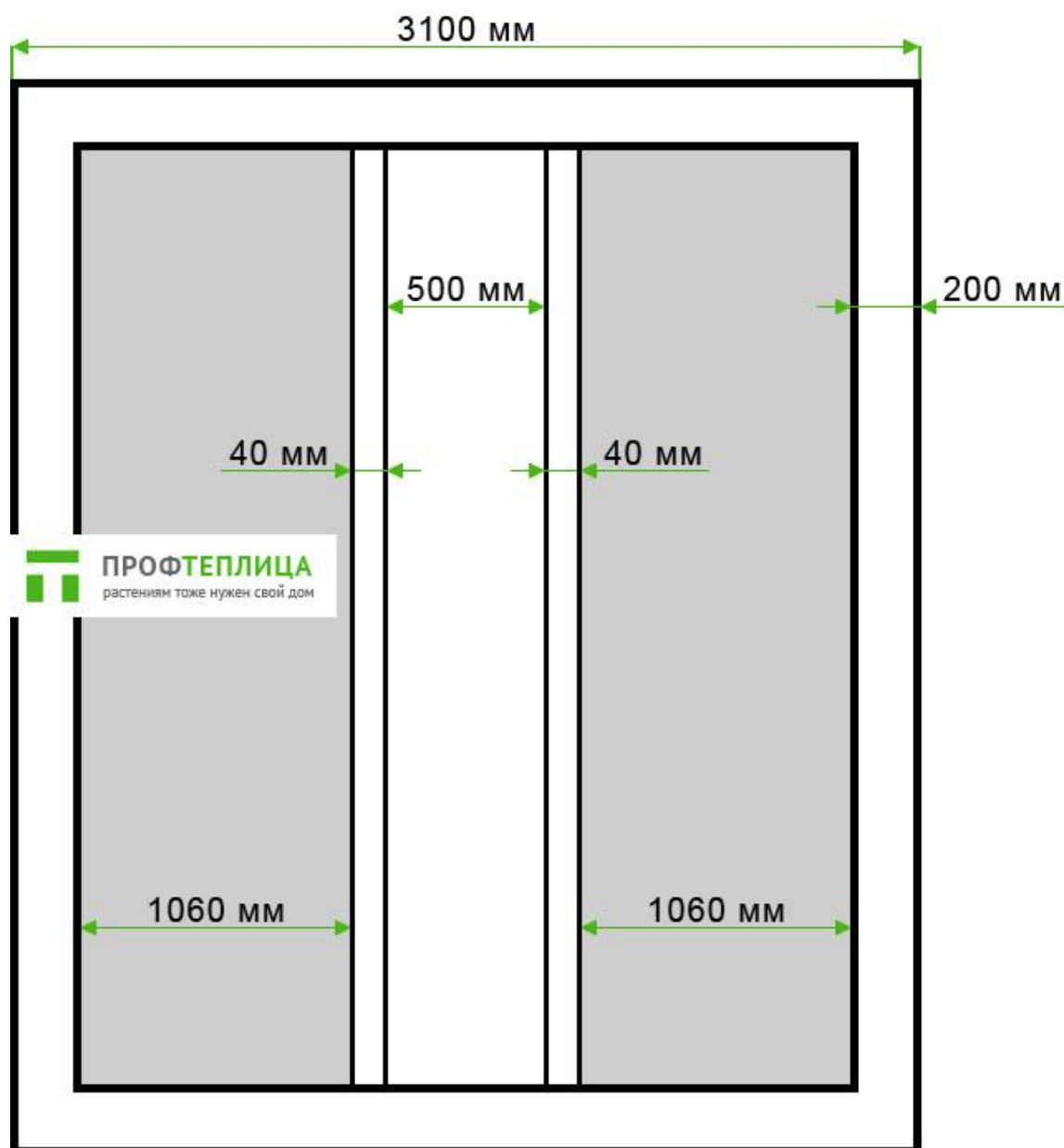
Вариант внутренней планировки теплицы «АСГ-16» (вид сверху)
