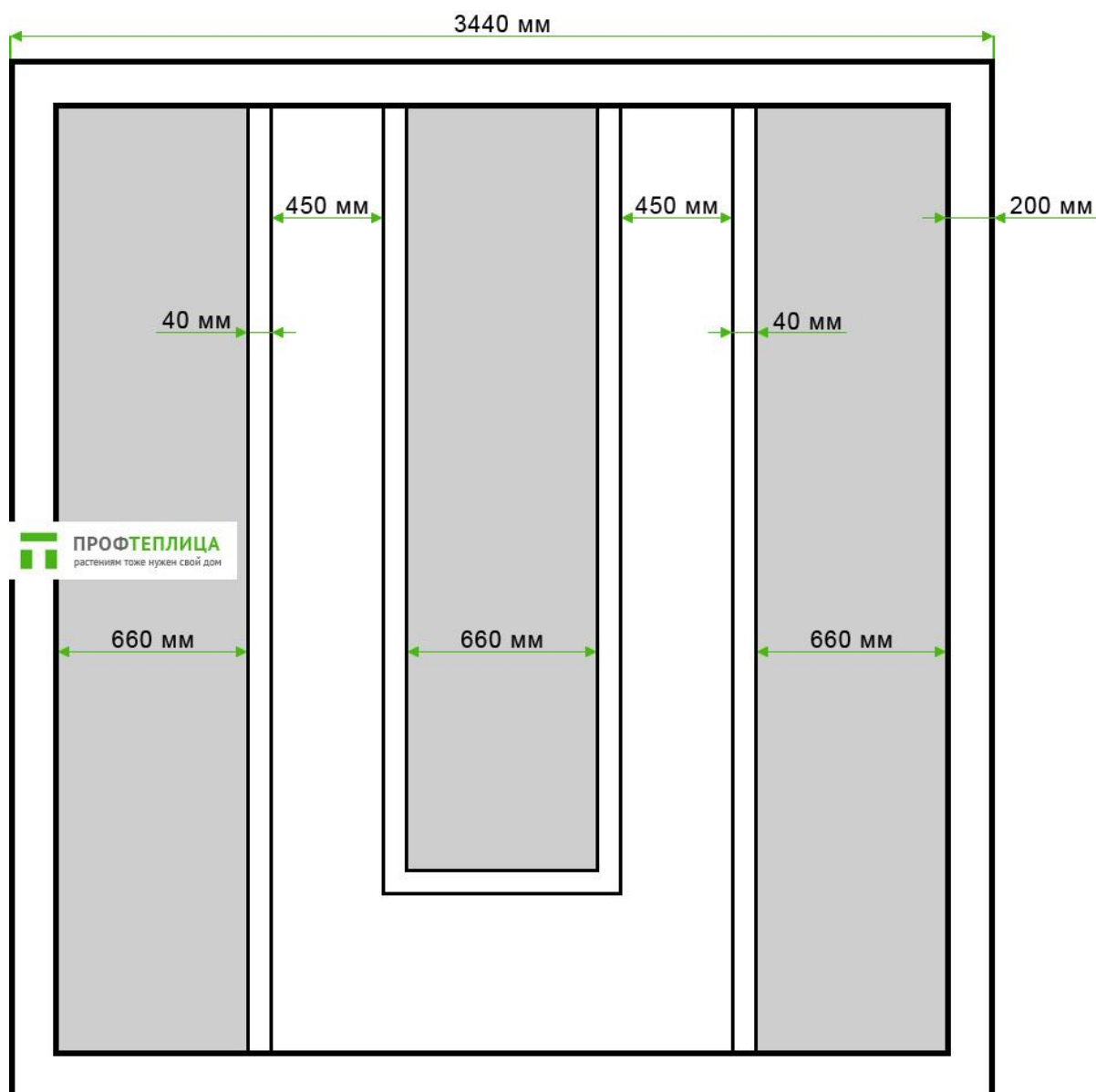
Вариант внутренней планировки теплицы «АСГ-18» (вид сверху)
