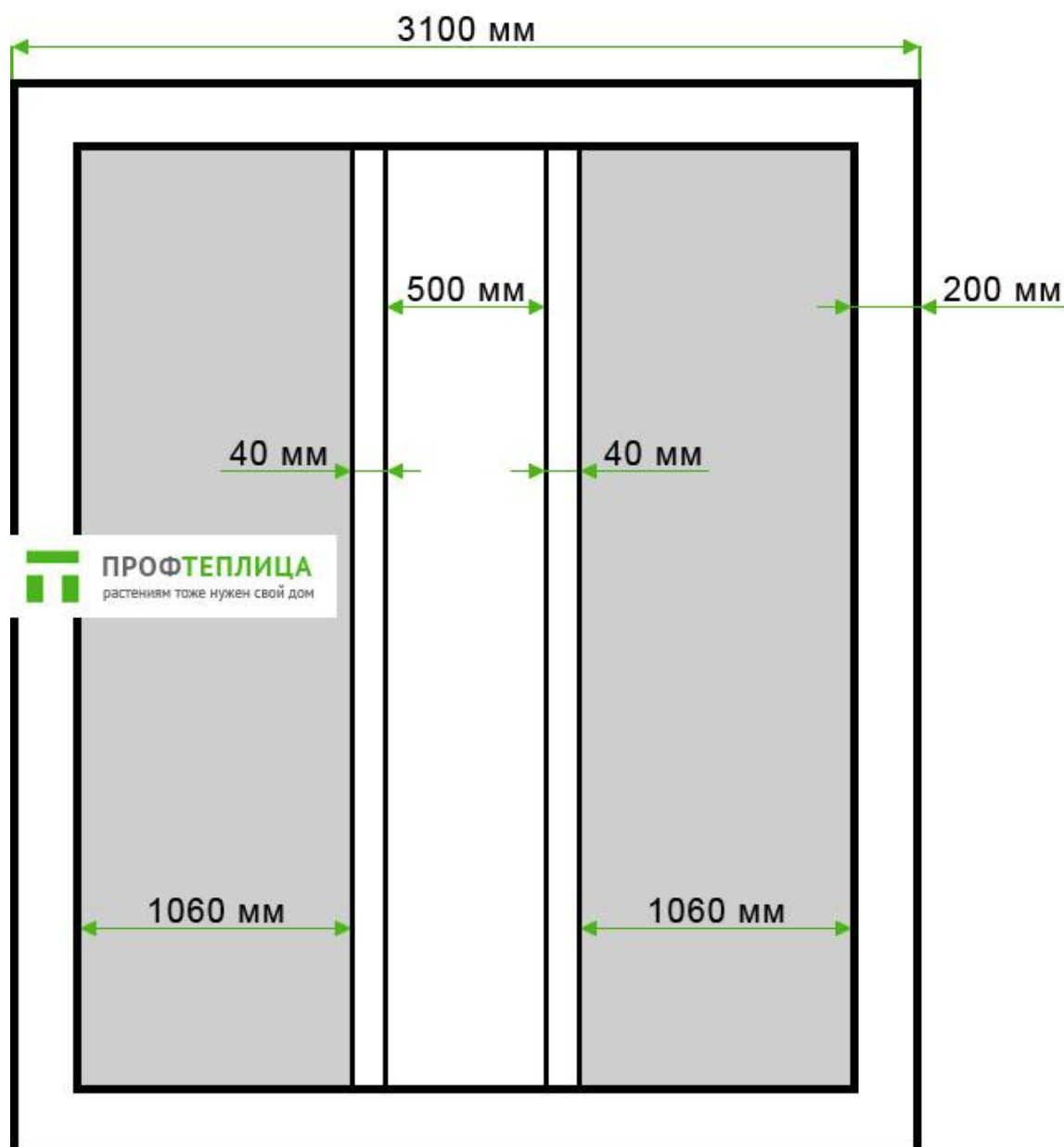
Вариант внутренней планировки теплицы «АСГ-20» (вид сверху)
