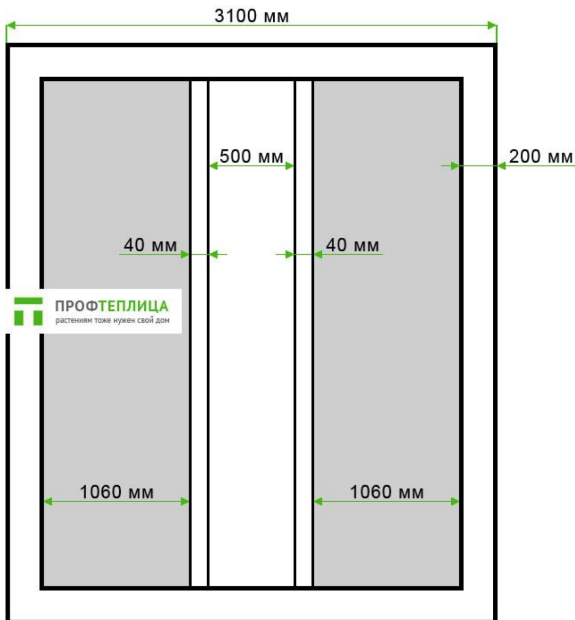
Вариант внутренней планировки теплицы «АСГ-9» (вид сверху)
